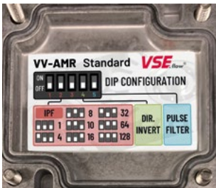
Abbildung 4: Vorverstärker-Peripherie
