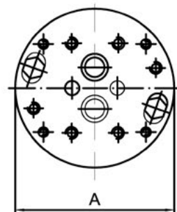
Ansicht X
