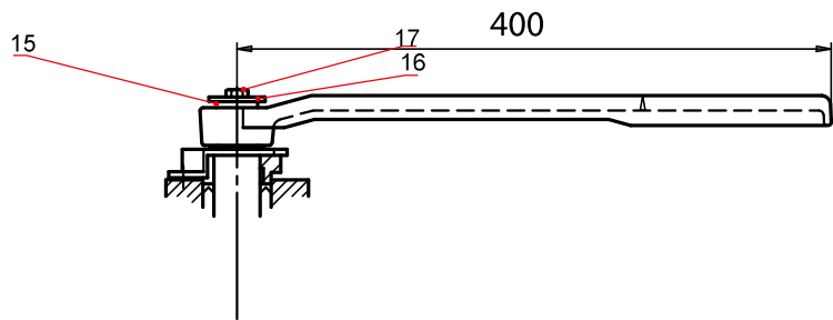
Handhebel bei DN 150 + DN 200 (Stah lackiertl) / handle at DN 150 + DN 200 (Steel painted)
