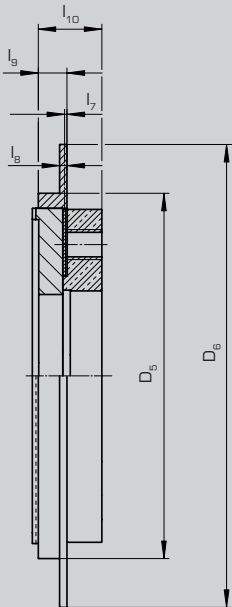
Bauform 6
