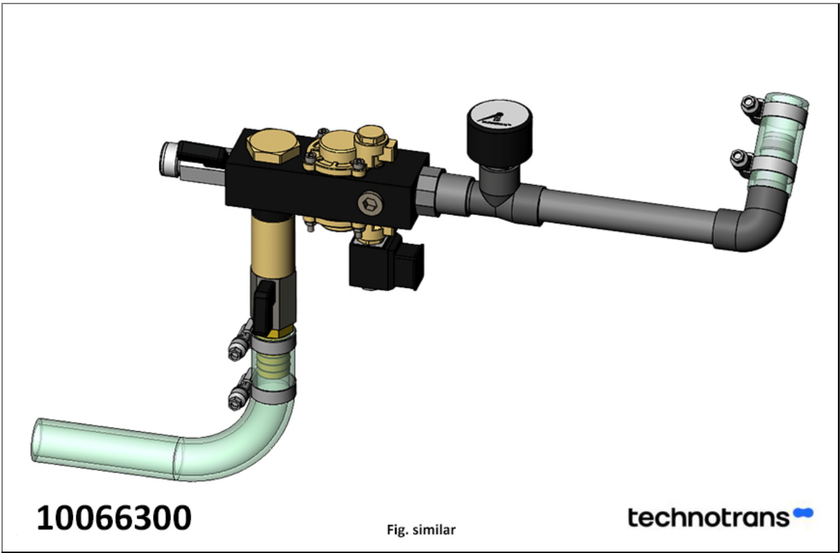
Fig.: / Abb.: Pipework / Verrohrung
