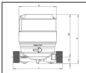
DN 15 laiton
