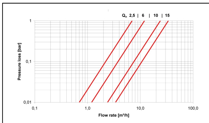
Druckverlustkurve
