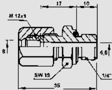
MAU 8 / Nst alle Maßangaben in mm
