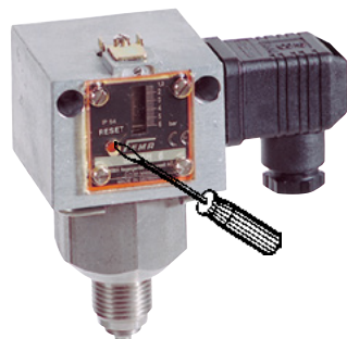
Druckbegrenzer mit interner Verriegelung
