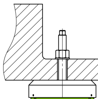
Einbaubeispiel
