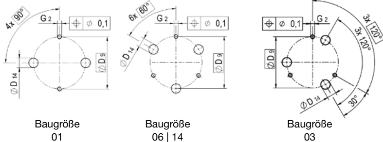
Bohrbild für Ankeraufnahme
