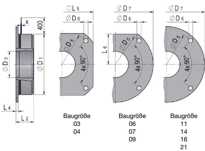
Typ 621 (flanschseitig montiert)
