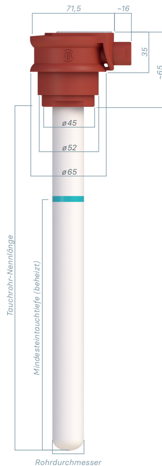
Kleinbadwärmer ROTKAPPE
