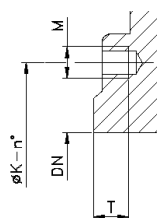
DN 900-1000
