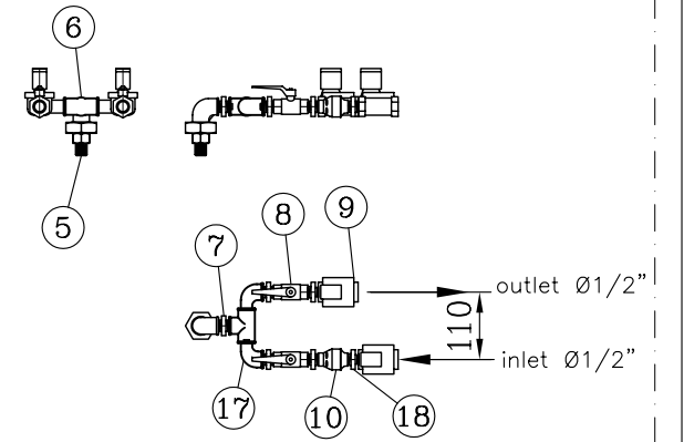
DETTAGLIO INGRESSO/USCITA AZOTO NITROGEN INLET/OUTLET DETAIL (4)
