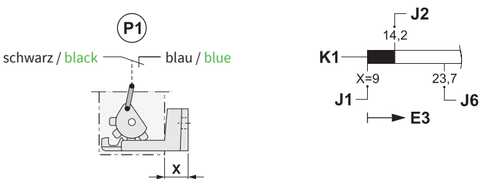
WZK10 (NC)
