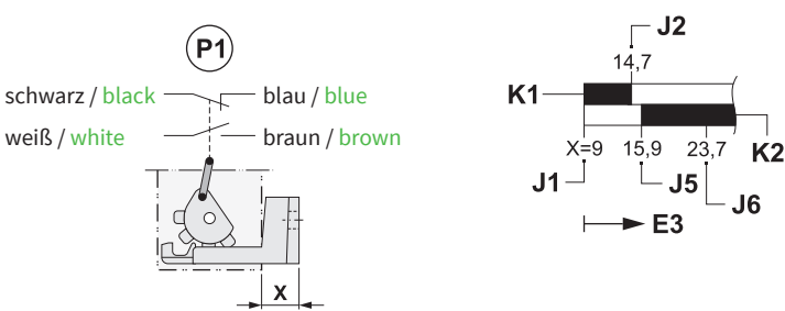
WZK11 (NC/NO)
