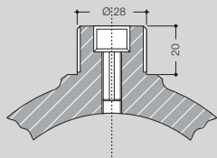
Valvola gas versione 2
