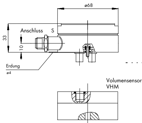
Zweifachaufnehmer
