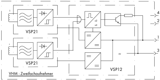
Blockschaltbild
