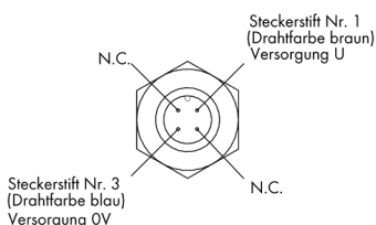
Steckerbelegung
