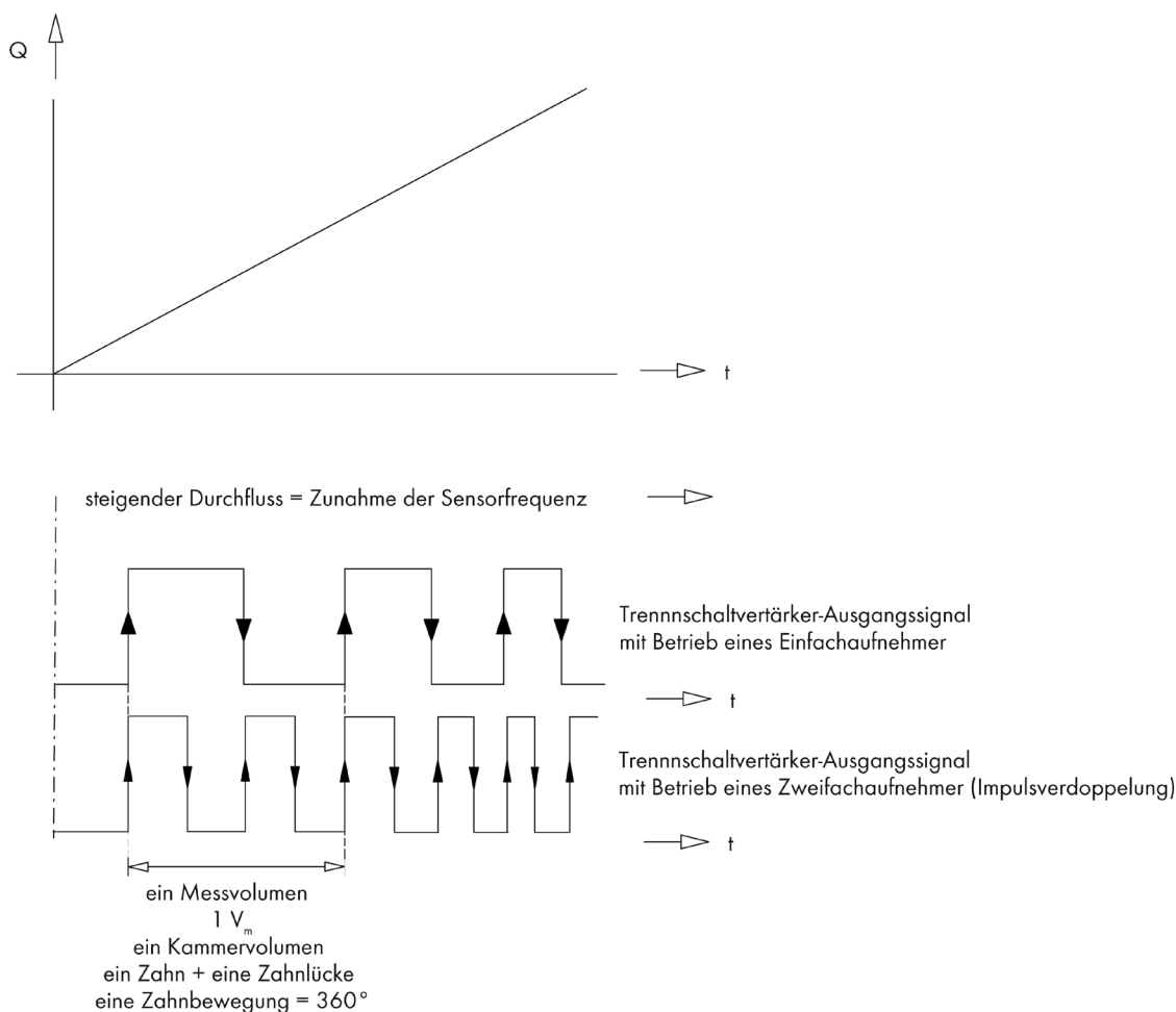
Abbildung 7: Signalausgabe
