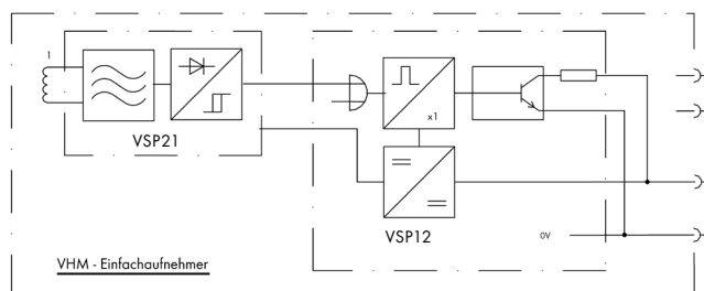
Blockschaltbild
