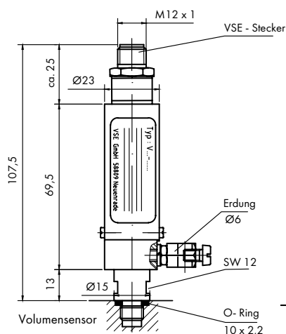
Einfachaufnehmer
