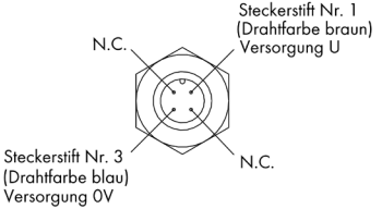
Steckerbelegung
