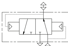
ANSI Symbol
