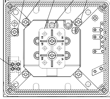
Teilschnitt D-D Maßstab 1:1
