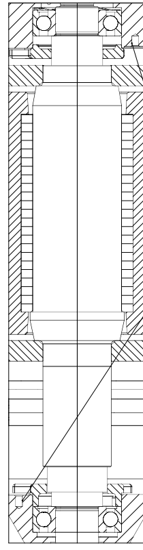
Teilschnitt B-B Maßstab 1:1
