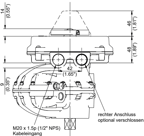
Direktmontage: Antriebsgr. 07, 08, 09, 10
