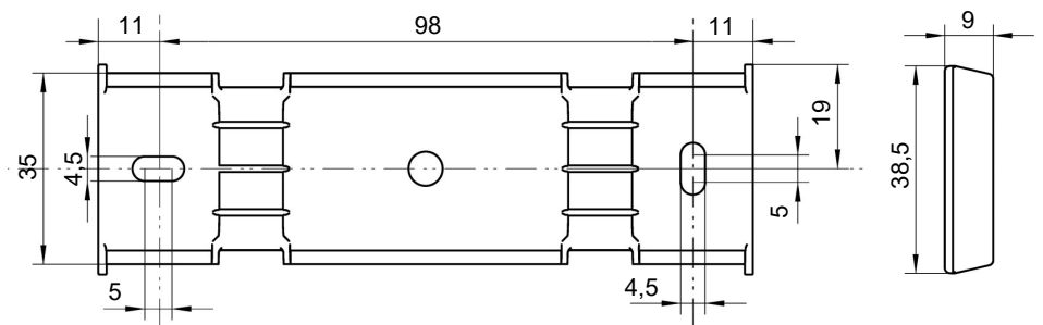
Abb. 6: Montageschiene
