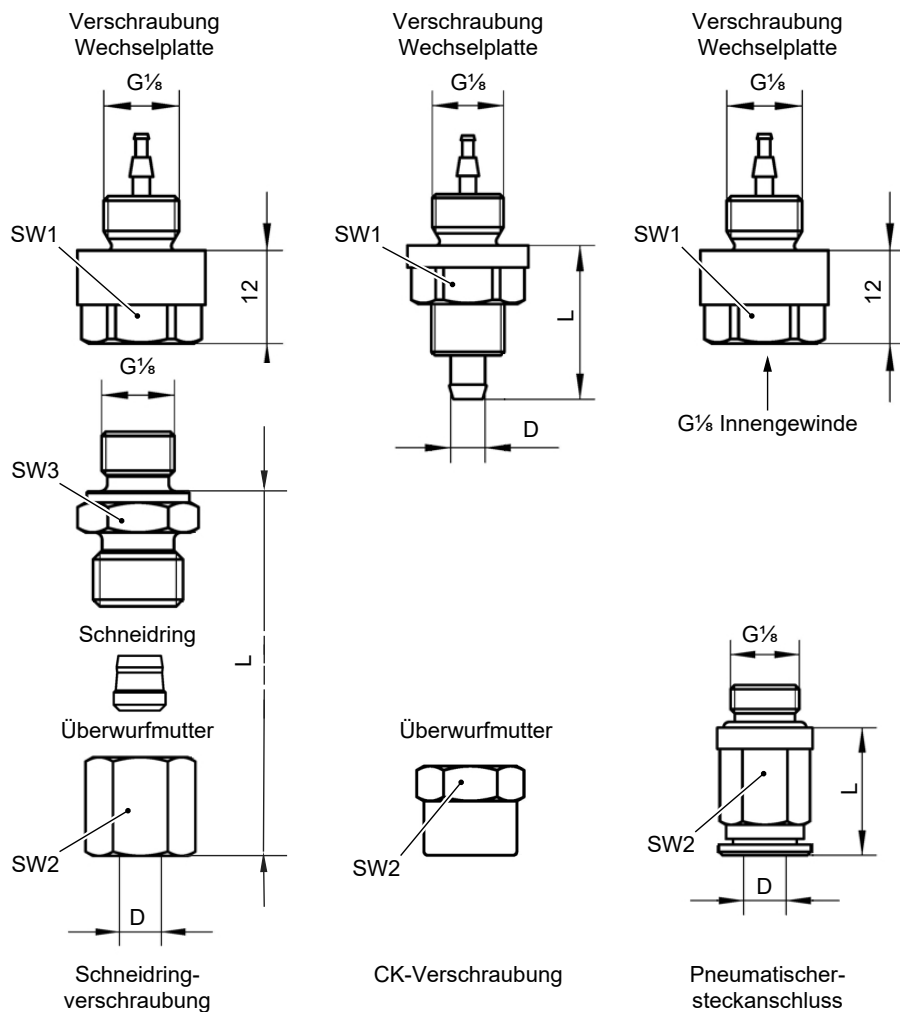
Abb. 7: Prozessanschluss Optionen
