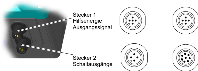
Abb. 3: Elektrische Anschlüsse
