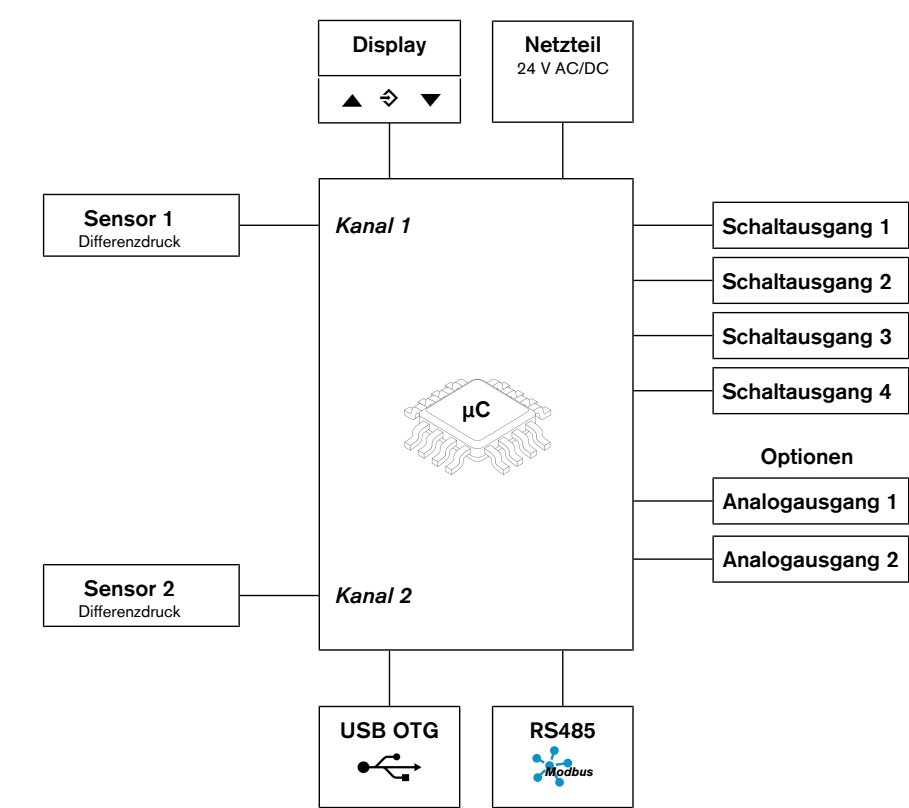
Abb. 1: Funktionsbild
