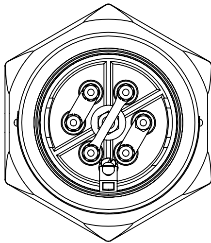
3 PHASE DELTA NO T-STAT
