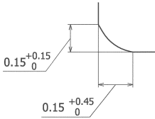
B部詳細図
