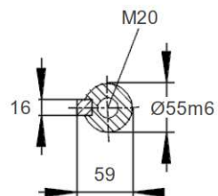
Welle A-Seite shaft DE
