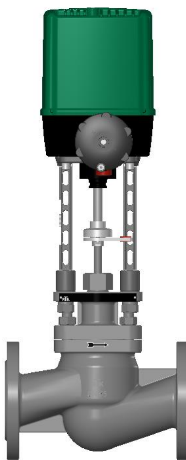
REact 30E/ DC mit Joch / with Yoke / avec joug
