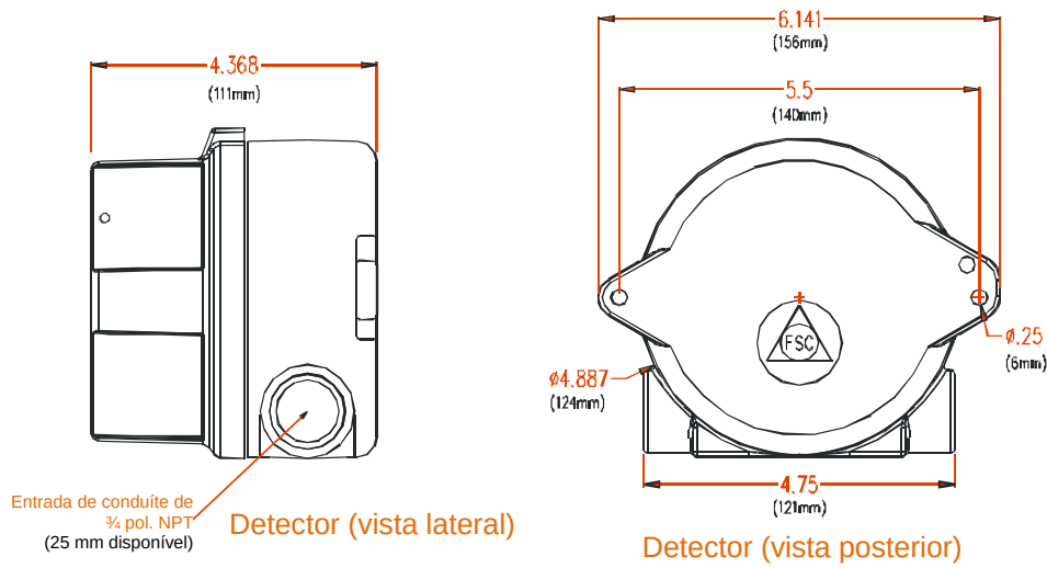
Figura 4-3 Descrição e dimensões do detector FS24X
