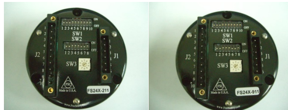
Figura 2-10 Disco dos detectores FS24X e FS24X-9, (vista posterior)
