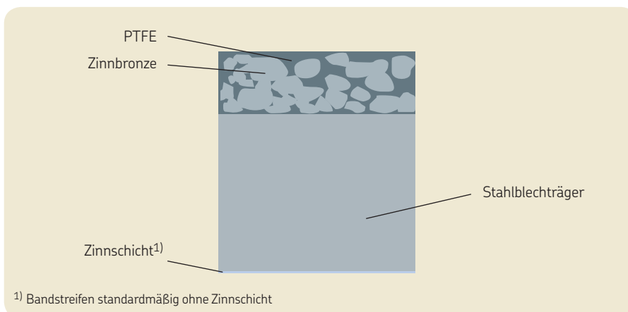
Querschnitt eines SKF PTFE Composite-Gleitlagers
