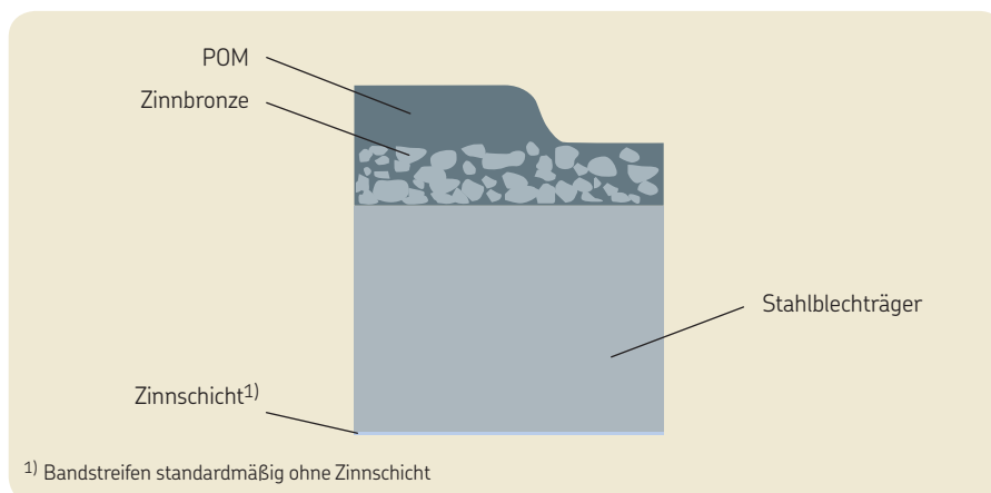
Querschnitt eines SKF POM Composite-Gleitlagers
