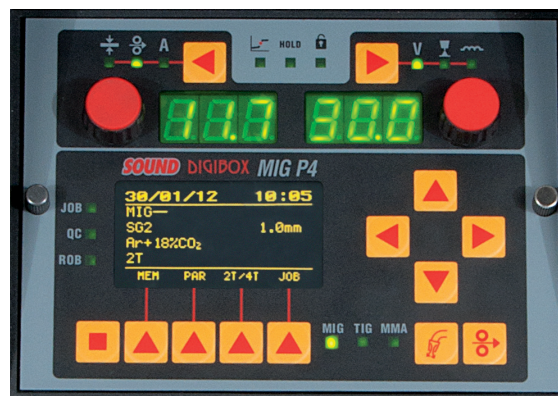
Neues Steuerpanel New control panel
