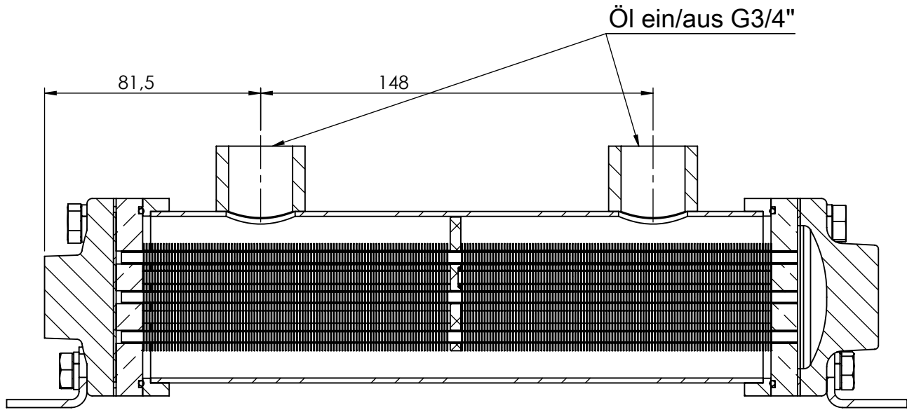
SCHNITT A-A MAßSTAB 1 : 2
