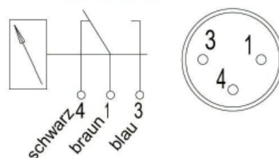
Anschlussbild:
