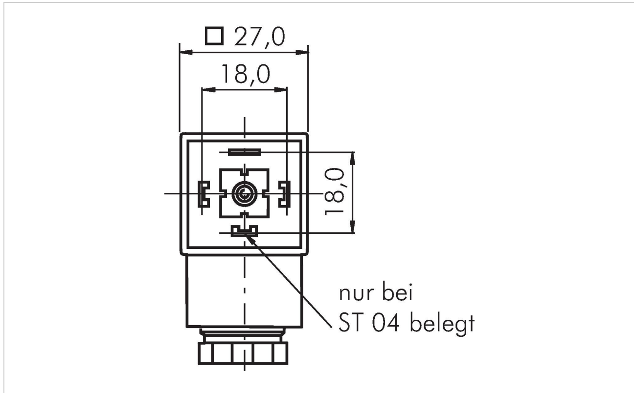
Zeichnung: Steckergröße 3 (DIN/EN-A)
