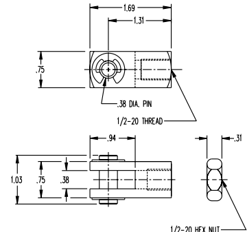
Piston Rod Clevis
