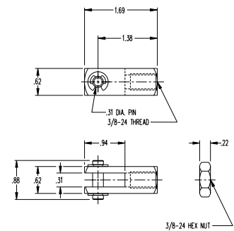
Rod Clevis
