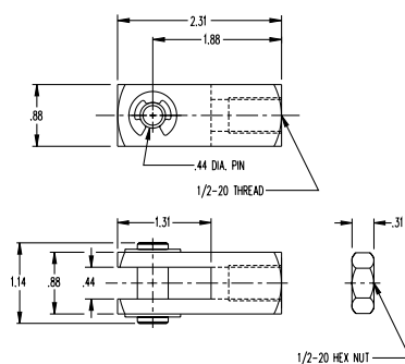
Rod Clevis
