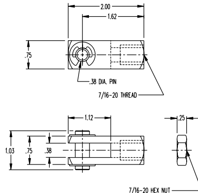
Rod Clevis
