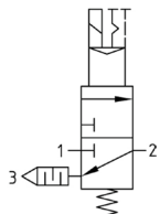
Schaltbild
