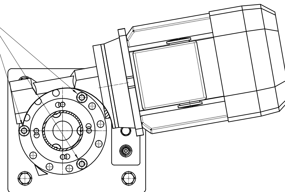
POSIZIONE DI MONTAGGIO GRUPPO DX CON COCLEA
