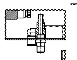
Sezione A-A
