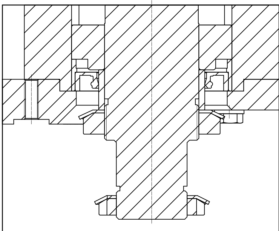
Dettaglio3 Scala 1:1
