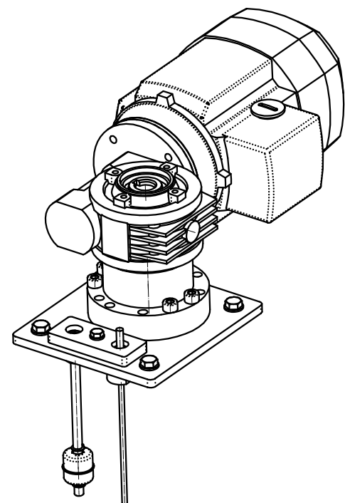
POSIZIONE DI MONTAGGIO GRUPPO SX SENZA COCLEA
