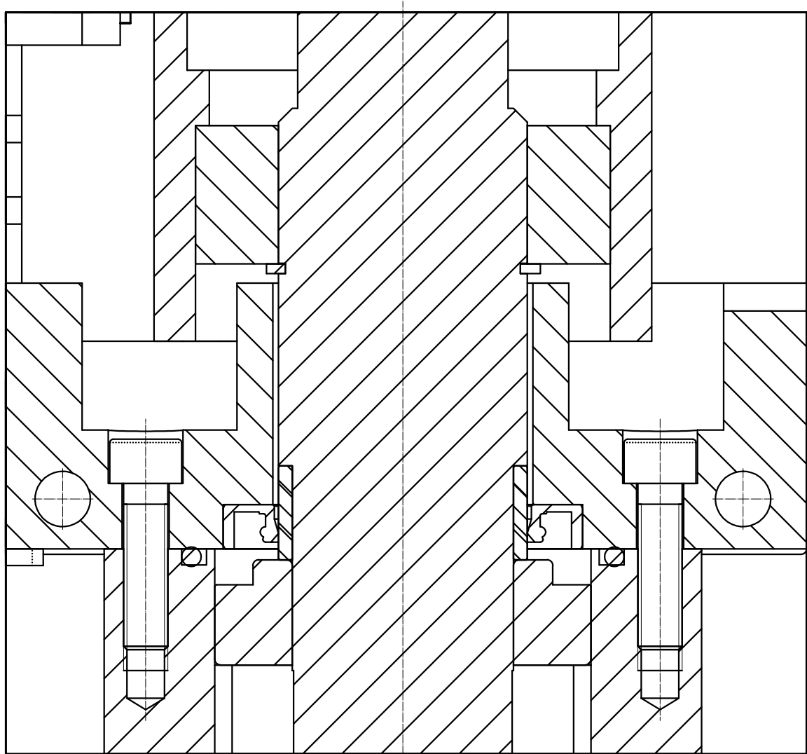
Dettaglio2 Scala 1:1
