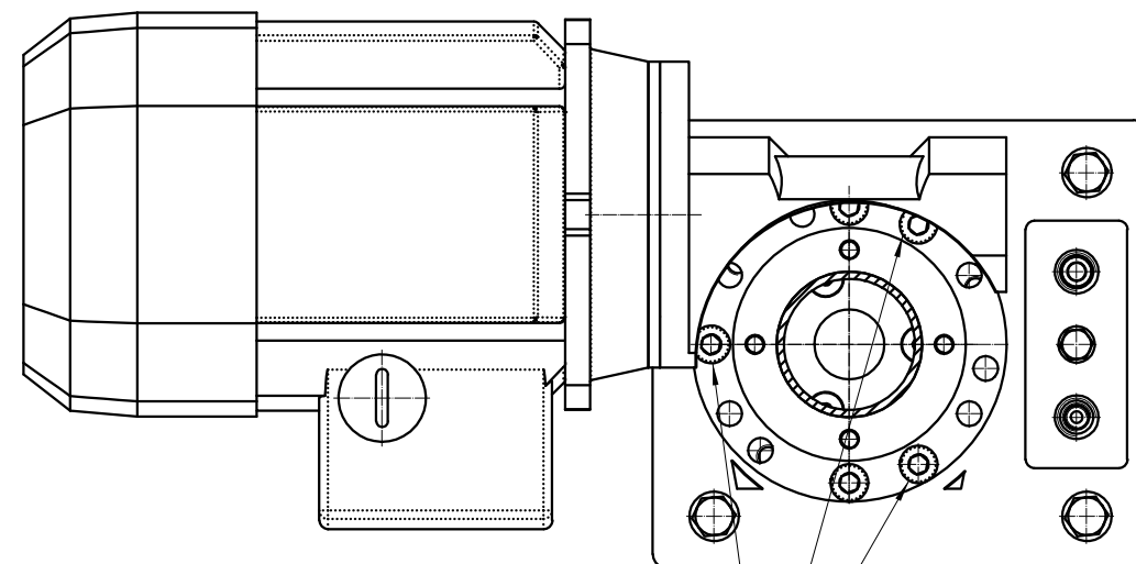
POSIZIONE DI MONTAGGIO GRUPPO DX SENZA COCLEA
