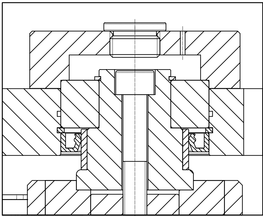
Dettaglio1 Scala 1:1
