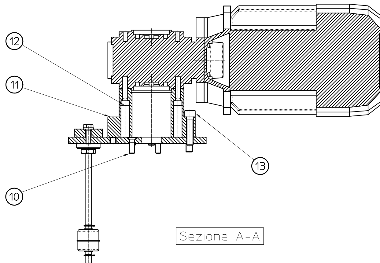
POSIZIONE DI MONTAGGIO GRUPPO SX SENZA COCLEA
