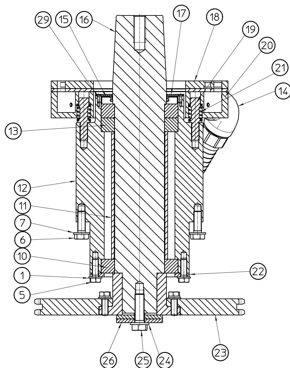
Sezione A-A
