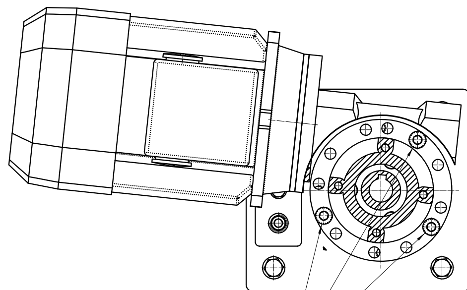
POSIZIONE MONTAGGIO GRUPPO SX CON COCLEA
