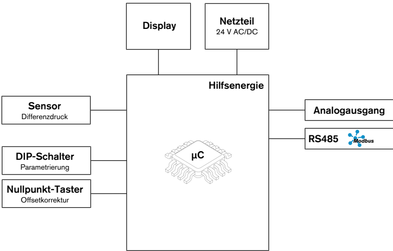
Abb. 1: Funktionsbild
