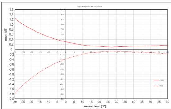
Abb. 1. Typischer Temperaturgang EFD-0691
