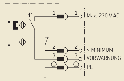
Kontaktdarstellung für max. gefüllten Behälter
