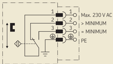
Kontaktdarstellung für max. gefüllten Behälter
