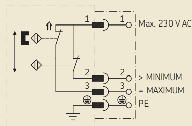
Kontaktdarstellung für max. gefüllten Behälter
