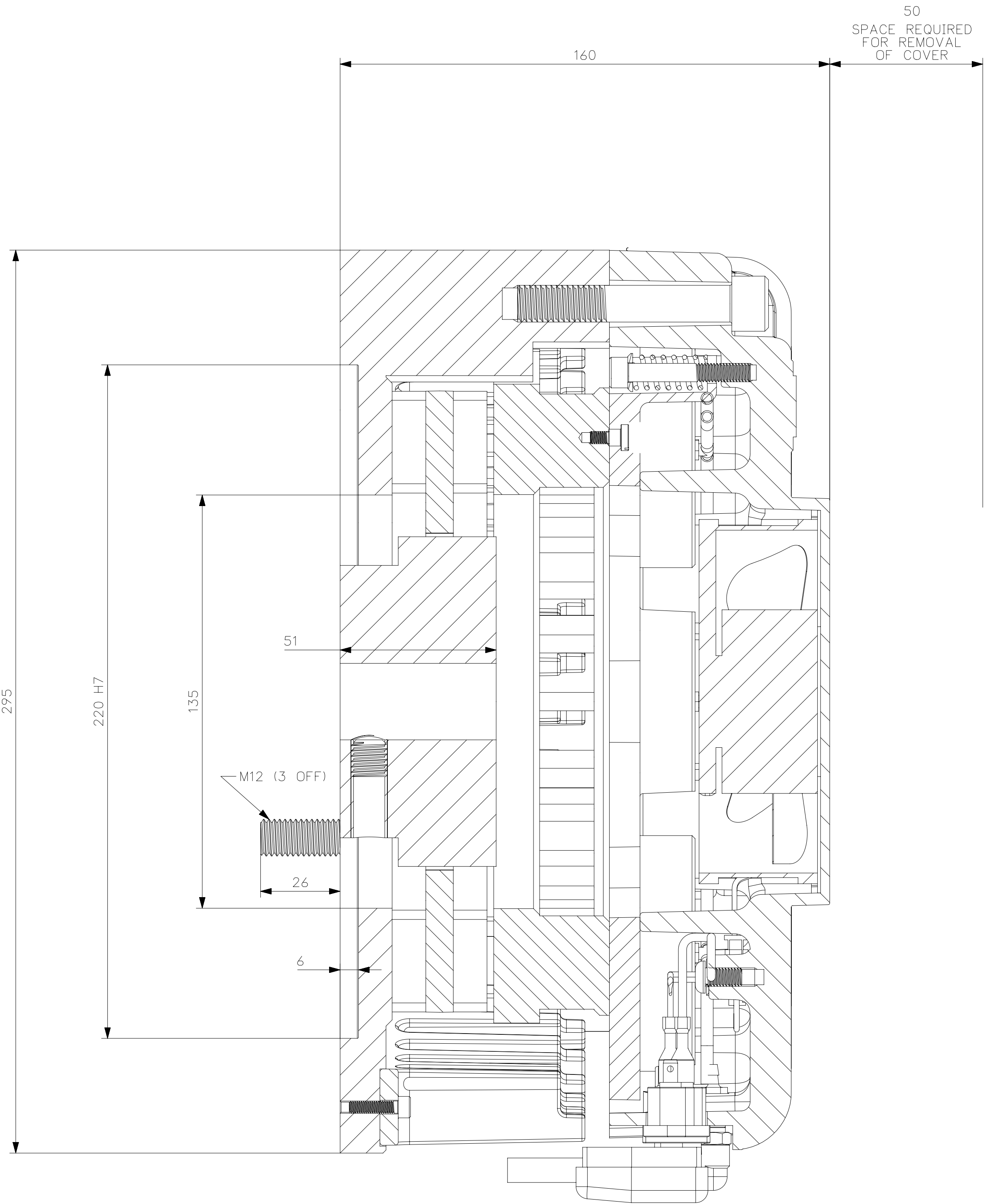
SECTION D-D
