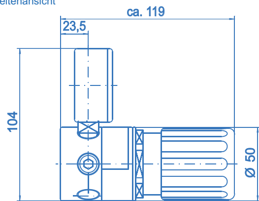
Seitenansicht
