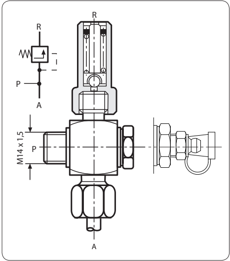
Druckbegrenzungsventil (DBV)
