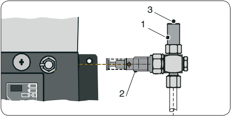
Anschluss Druckbegrenzungsventil
