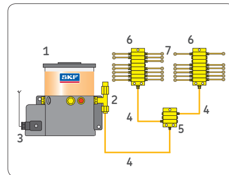
Beispiel einer Progressivanlage mit KFG Pumpenaggregat
