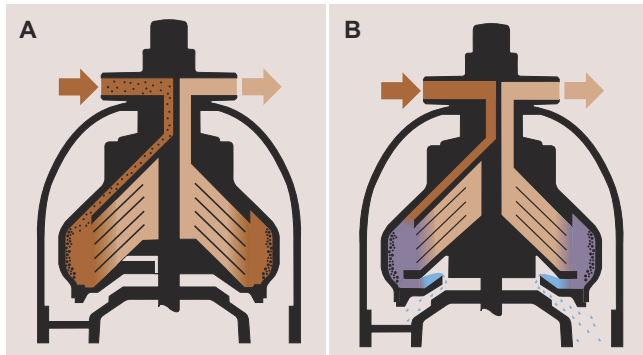
A. Clarifier
