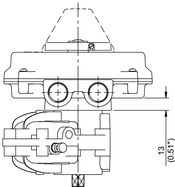
Direktmontage mit zusätzlicher Adapterplatte, zusätzl. Gewicht: 0.04 kg / 0.09 lb
