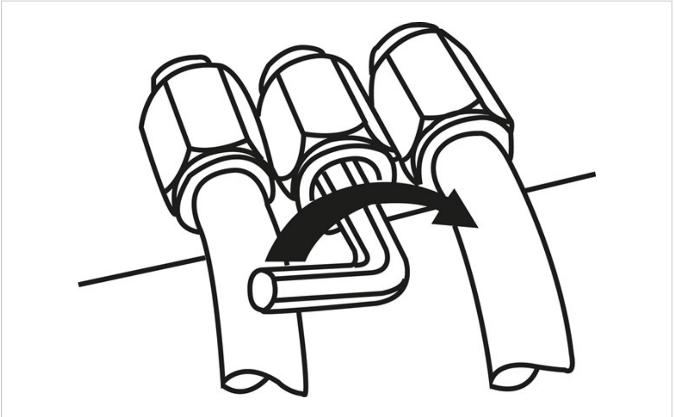
Drawing: Steckverschraubung durch Innensechskant montierbar
