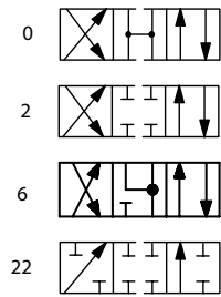
DG4V-3(S)-*NV
