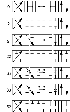
DG4V-3(S)-*CV
