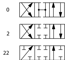
DG4V-3(S)-*ALV
