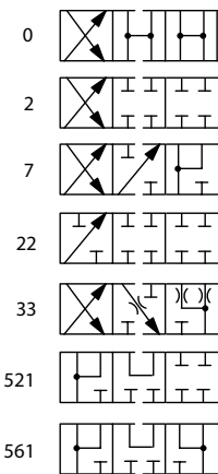
DG4V-3(S)-*BV
