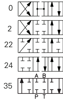
DG4V-3(S)-*BV
