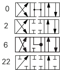
DG4V-3(S)-*NV
