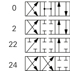
DG4V-3(S)-*ALV
