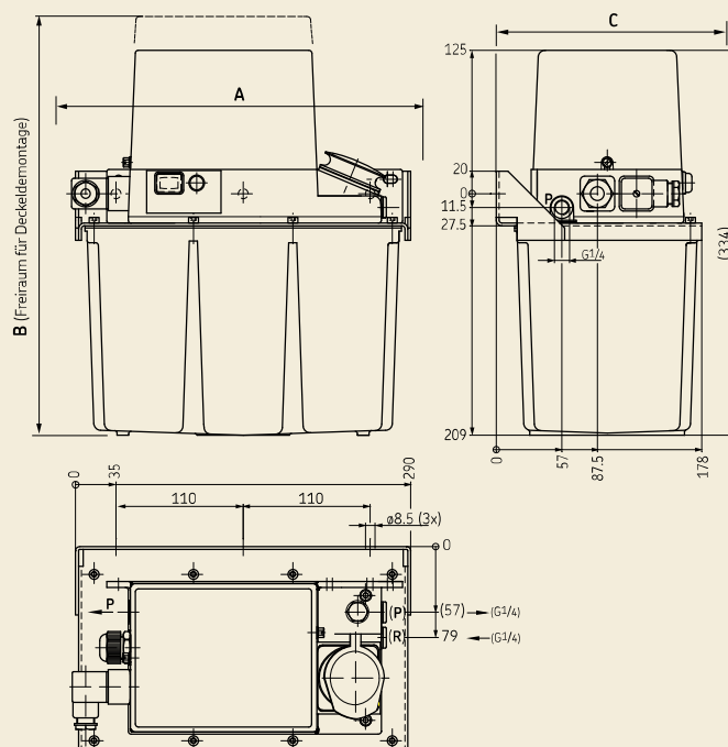
MKx-Aggregat mit 6 Liter Kunststoffbehälter für Öl und Fließfett
