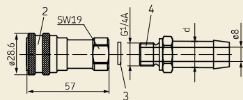
Befüllleinrichtung mittels Schnellkupplung
