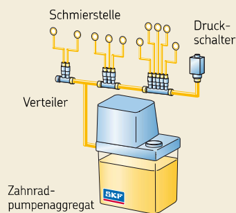
Nachschmierverteilersystem
