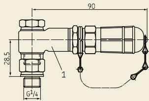
Befüllleinrichtung komplett mit Schwenkverschraubung
