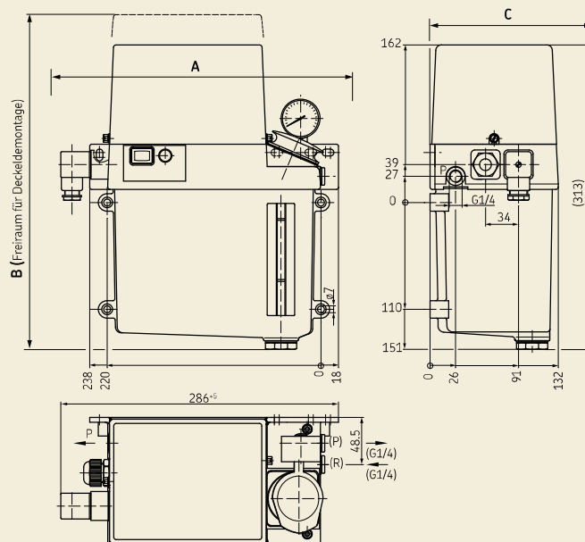
MKx-Aggregat mit 3 Liter Metallbehälter für Öl und Öl+Luft
