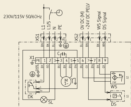
Schaltbild 3
