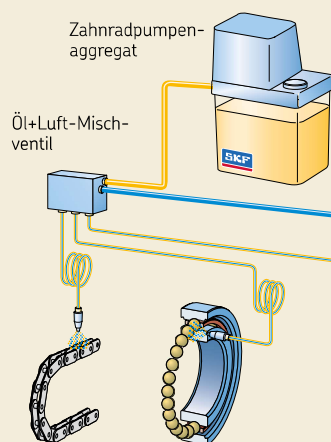
Öl+Luft-System
