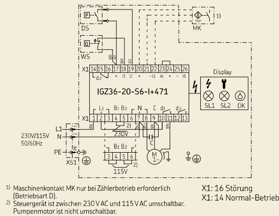
Schaltbild 6
