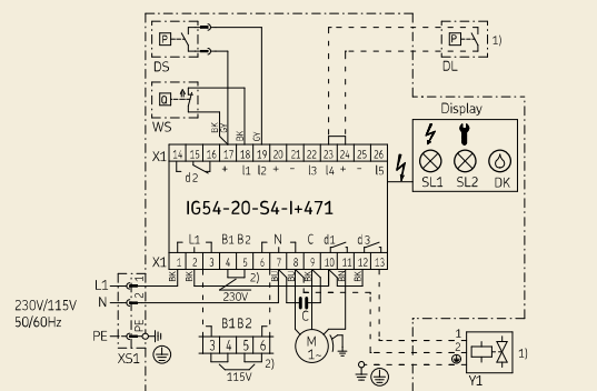
Schaltbild 7
