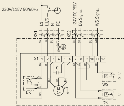
Schaltbild 1
