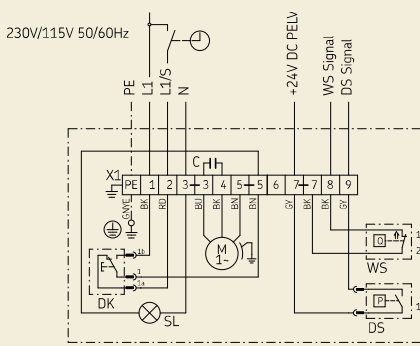
Schaltbild 4
