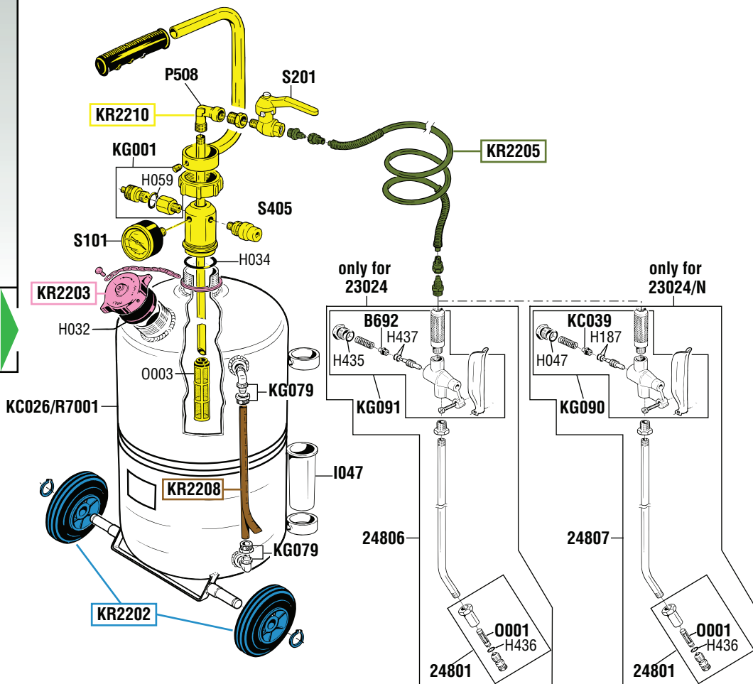
NEBULIZZATORE CARRELLATO INOX VERNICIATO CON SERBATOIO DA 24 l PAINTED STAINLESS STEEL WHEEL-MOUNTED PRESSURE SPRAYER WITH 24 l TANK
