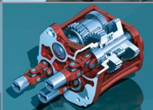
ZF-Servoplan PG Servogetriebe
