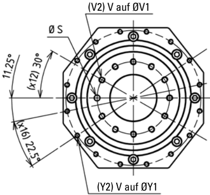
Baugröße 800
