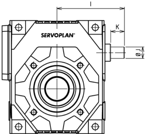
Baugröße 800
