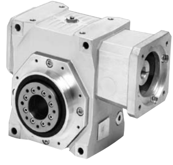
Abtrieb mit Roboterflansch nur Baugrößen (80 bis 800)
