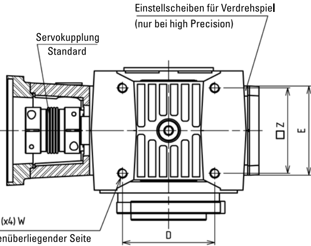
Baugröße 80,120 und 190
