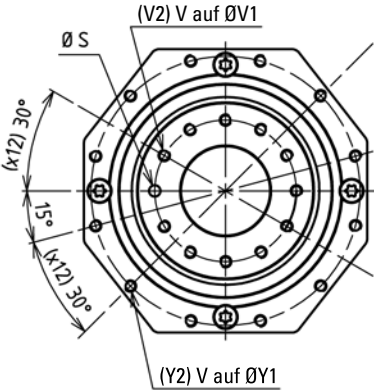
Baugröße 260 und 500
