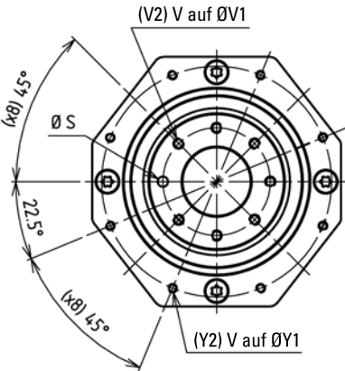
Baugröße 80,120 und 190
