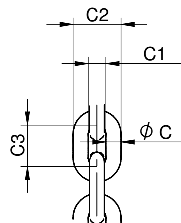
DETTAGLIO Y2
