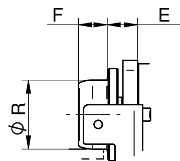
DETTAGLIO Y3
