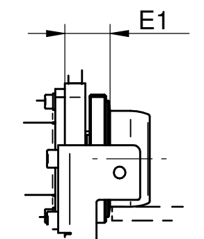
DETTAGLIO Y4
