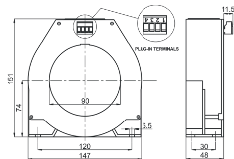
TDB090... kg. 0,74
