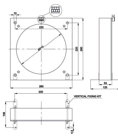
TDB210... kg. 1,9
