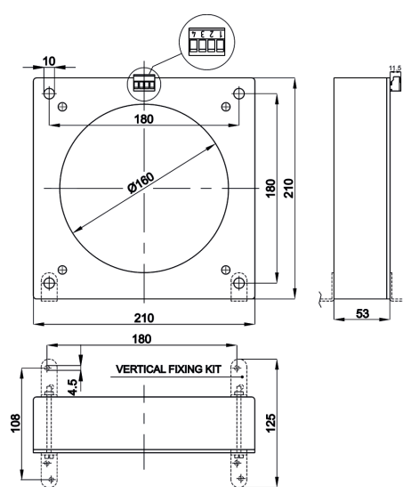
TDB160... kg. 1,5
