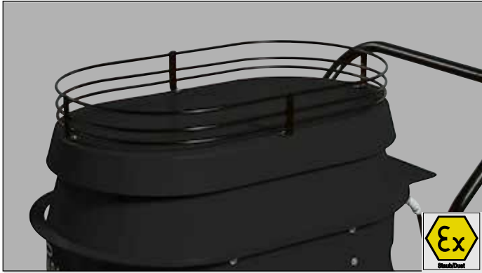
Zubehörkorb für R01 A Stahlrohr pulverbeschichtet, schwarz, Montage auf der Schallhaube L - 578 mm, B - 324 mm, H - 70 mm Art-Nr: 16956
