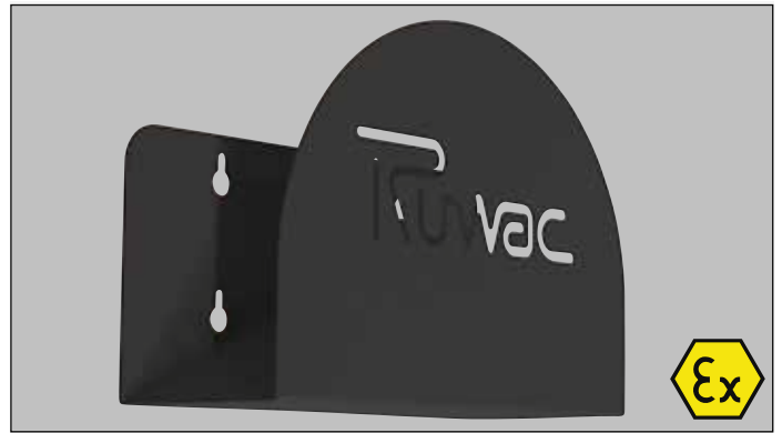
Schlauchhalter, Stahlblech, pulverbeschichtet, Montage an der Wand L - 330 mm, B - 123 mm, H - 238 mm, inkl. Befestigungsmaterial Art-Nr: 12080 (rot) Art-Nr: 12081 (schwarz)
