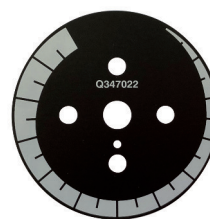
QUADRANTE tipo Q3 Ø mm. 60 - interasse Ø 28
